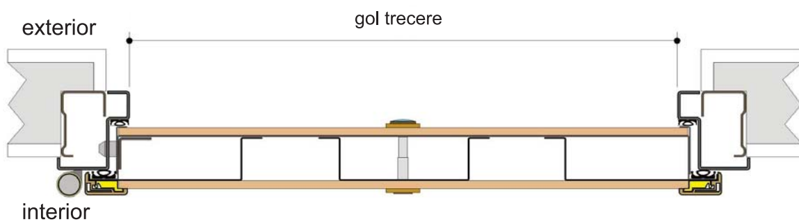
Sectiune foaie de usa
